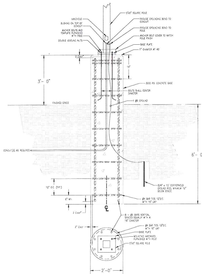
1 LIGHTING POLE BASE DETAIL E000 N.T.S.
